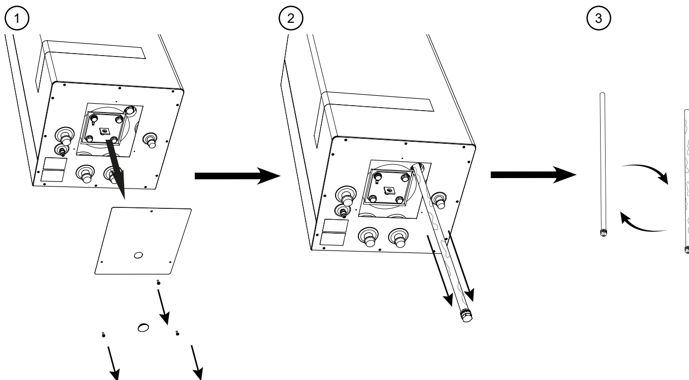
Fig.20 Udskiftning af magnesiumanode i beholderne QM 100, QM 150.
