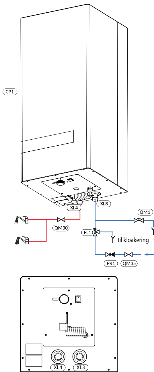
Fig.10 Principtegninger for QME.
