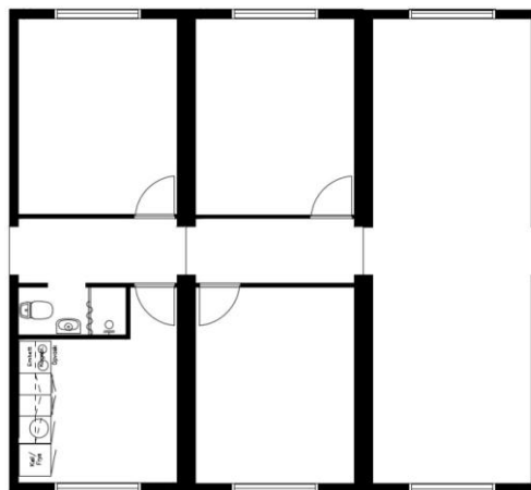
Systemmodul 50 + 51 + 52
